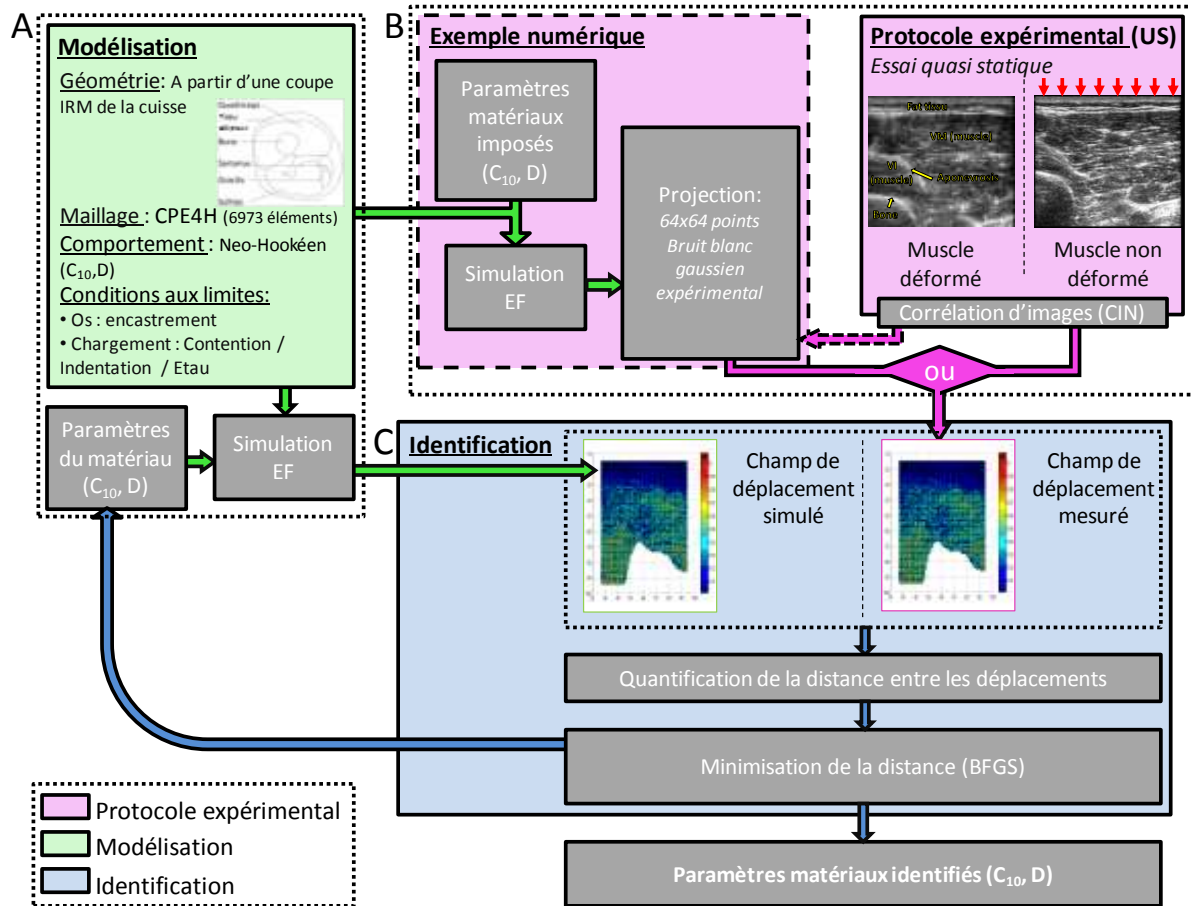
Figure II.1 : Schéma de la démarche d'identification globale par approche inverse de type FEMU (Finite Element Model Updating) développée dans cette thèse. (A) Modélisation, (B) Protocole expérimental, (C) Identification.
