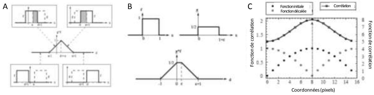
Figure II.10 : (A) Fonction d'inter-corrélation entre deux fonctions identiques. La valeur h(\Delta) est maximisée en \Delta=u . (B) Fonction d'inter-corrélation entre deux fonctions déformées l'une par rapport à l'autre d'une quantité \varepsilon . (C) Fonction d'inter-corrélation discrète entre deux fonctions sinusoïdales échantillonnées [Hild et Roux, 2008].
