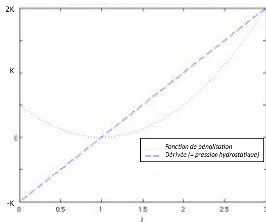
Figure I.13 : Evaluation de la fonction de pénalisation : U(J) = \frac{K}{2}(J-1)^2 (\dots) et de sa dérivée (---) en fonction du paramètre scalaire J .
