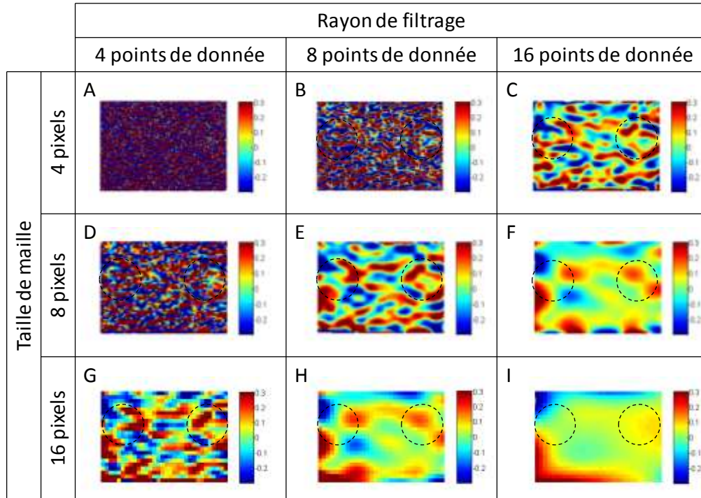
Figure III.12 : Cartographies du champ de déformation horizontal ( \varepsilon_{xx} ) en fonction de la taille de maille (exprimée en pixels) et de la taille du rayon de filtrage de valeurs respectives de : (A) 4, 4 (B) 4, 8 (C) 4,16 (D) 8, 4 (E) 8, 8 (F) 8, 16 (G) 16, 4 (H) 16, 8 (I) 16, 16.
