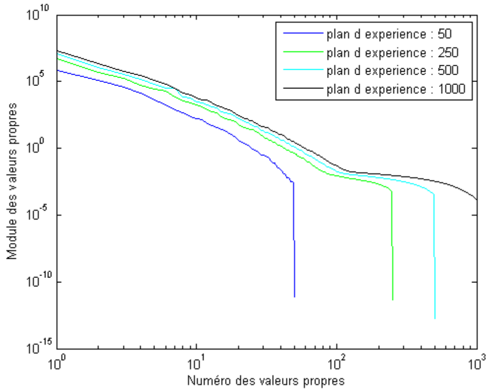
Figure III.23 : Module des valeurs propres évaluées lors de la POD pour des plans d'expérience de 50, 250, 500 et 1000 tirages par hypercube latin des jeux de 10 paramètres.
